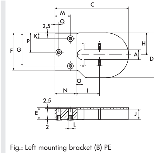
Fig.: Left mounting bracket (B) PE
