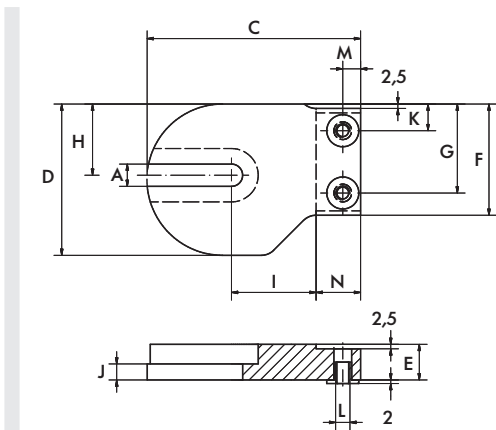
Fig.: Right mounting bracket (A) PE
