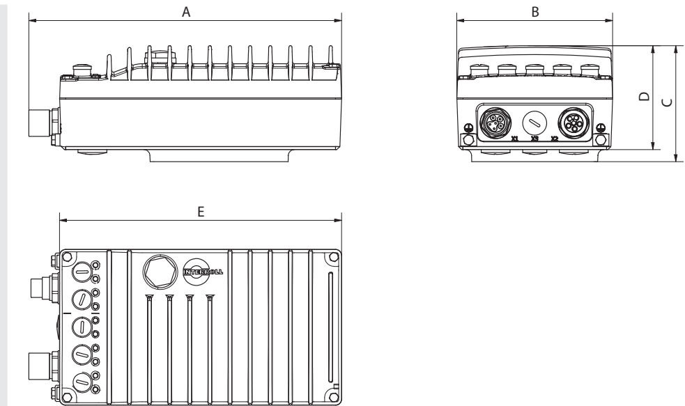
Fig.: FC 1000, motor-mounted, size 1 & 2
