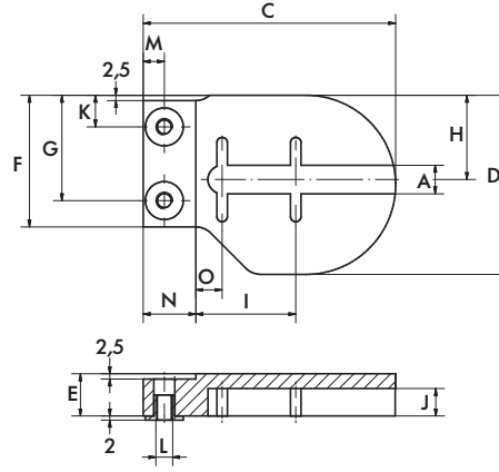
Fig.: Left mounting bracket (B) PE
